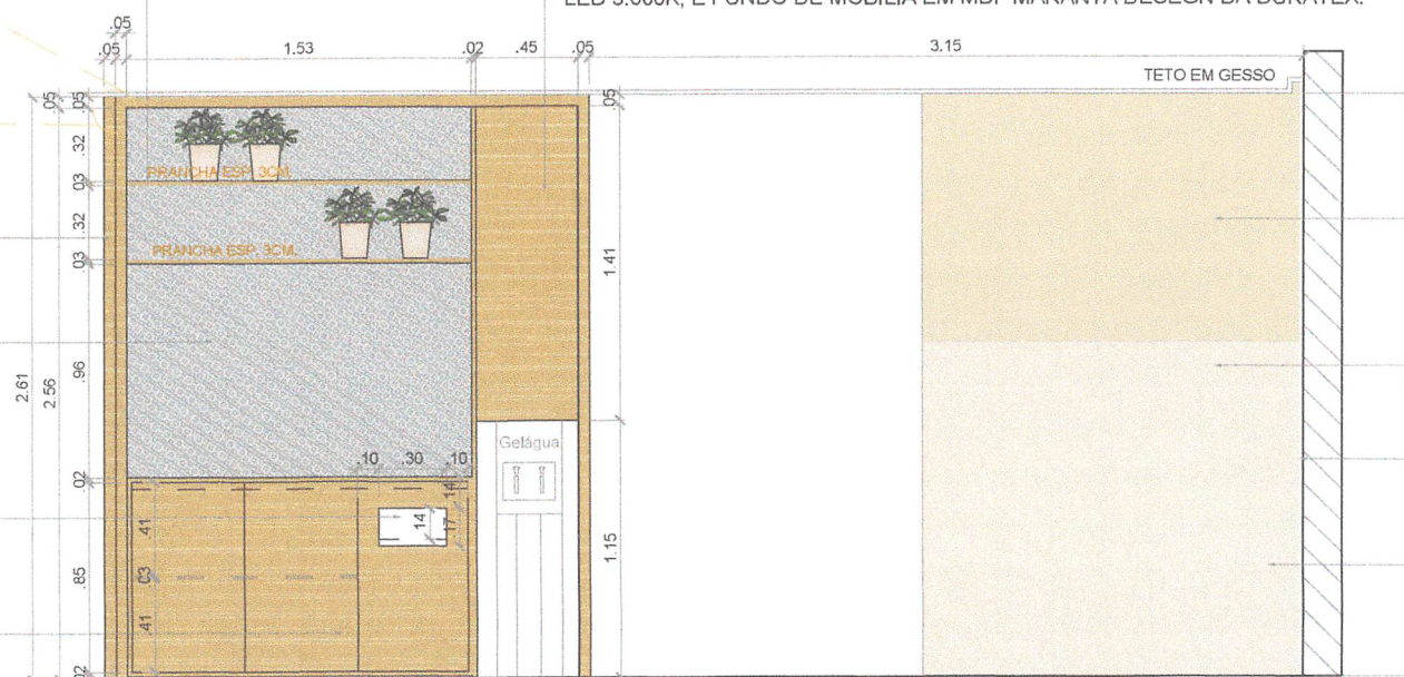
Corte CC - Recepção CDI ESCALA: 1/25
