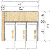
Corte CC - Balção ESCALA: 1/25
