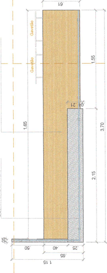
Planta Baixa - Balção ESCALA: 1/25
