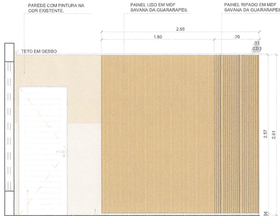
Corte BB - Recepção CDI ESCALA: 1/25
