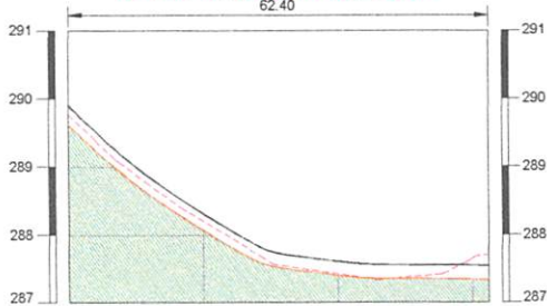
Perfil Longitudinal Escala: H.....1/5.000 V.....1/500
