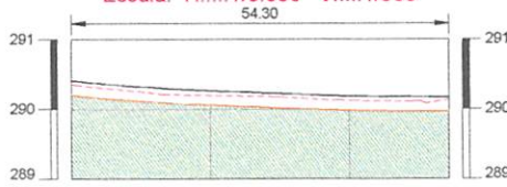
Perfil Longitudinal Escala: H.....1/5.000 V.....1/500
