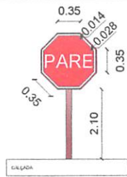
PLACA DE SINALIZAÇÃO ESCALA SEM ESCALA
