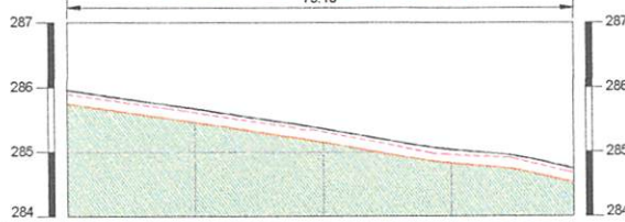
Perfil Longitudinal Escala: H.....1/5.000 V.....1/500
